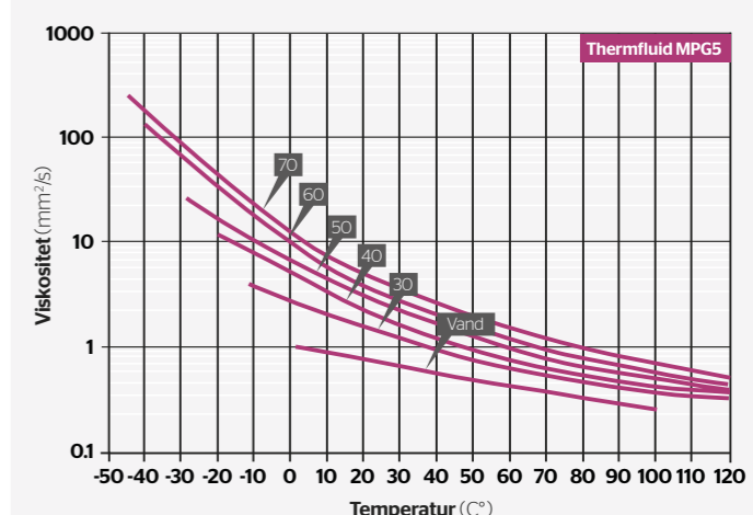
Kinematisk viskositet for THERMFLUID MPG5 i vand.
