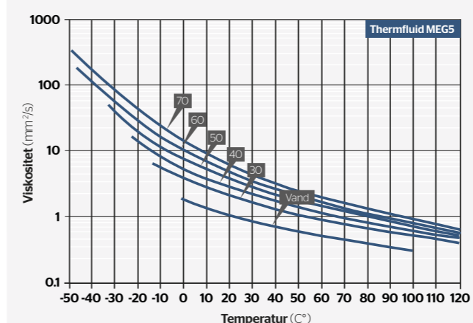
Kinematisk viskositet for THERMFLUID MEG5 i vand.
